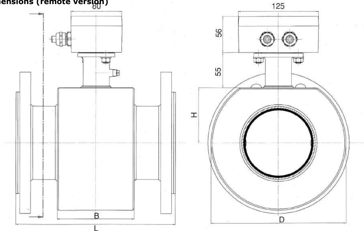
Fig. 10 Dimensions
